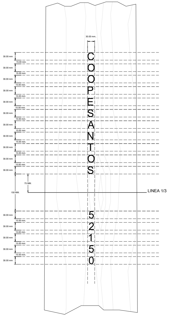
DETALLE AMPLIADO Y DIMENSIONES DE LAS LETRAS A IMPRIMIR EN EL POSTE DE MADERA
